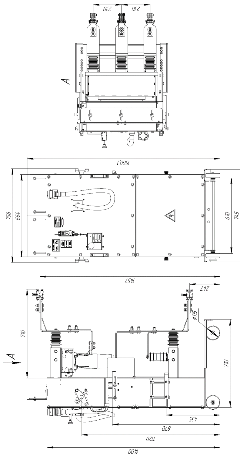
Рисунок Б.1 – Монтажный и габаритный чертеж выкатного элемента КЭПС-ВЭ КРУ 2-10 (вал вверх) без БУ
