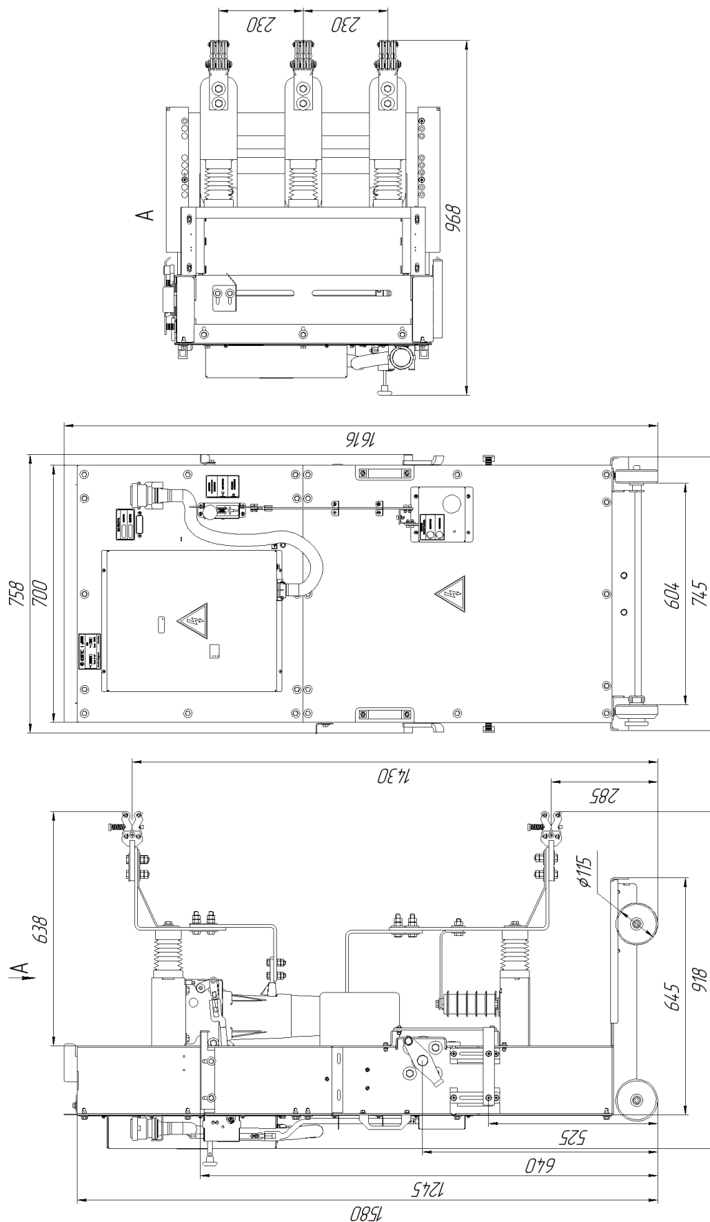
Рисунок А.2 – Монтажный и габаритный чертеж выкатного элемента КЭПС-ВЭ КРУ2-10 (вал внизу) с БУ
