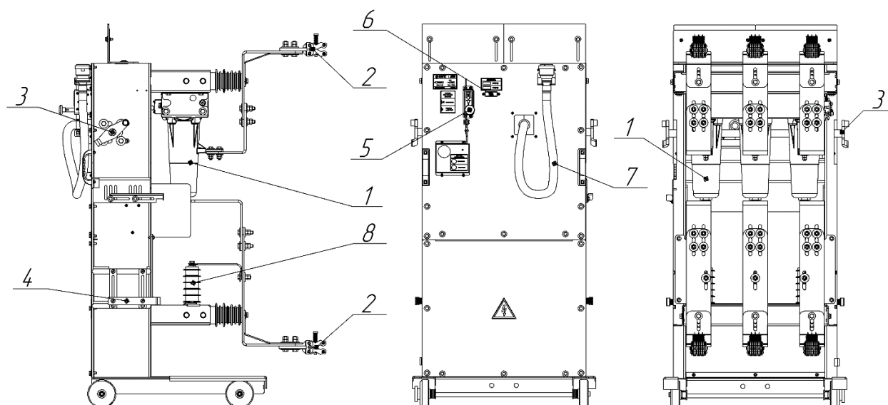
Рисунок 1.2 – Состав выкатного элемента КЭПС-ВЭ КРУ2-10 (КВЭ-10) вал вверх без БУ на щите
