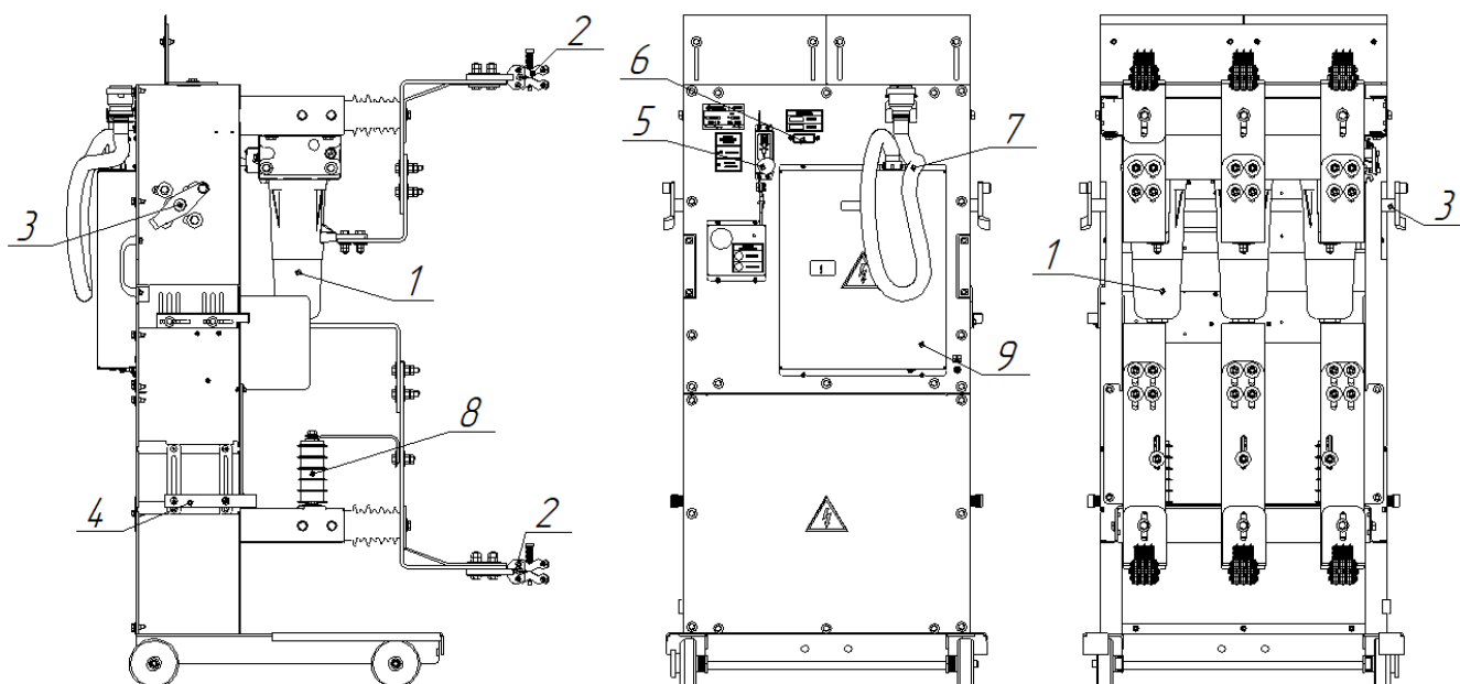
Рисунок 2.2 – Состав выкатного элемента КЭПС-ВЭ КРУ2-10 (КВЭ-10) вал вверху с БУ на щите
