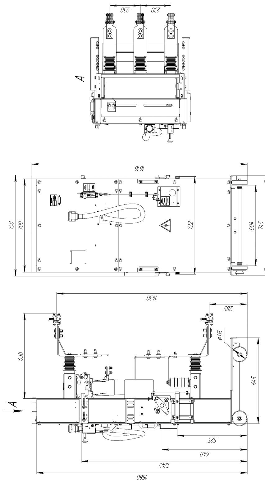
Рисунок А.1 – Монтажный и габаритный чертеж выкатного элемента КЭПС-ВЭ КРУ2-10 (вал внизу) без БУ
