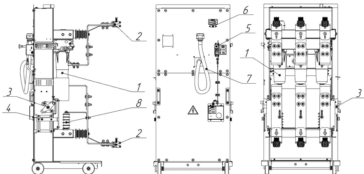
Рисунок 1.1 – Состав выкатного элемента КЭПС-ВЭ КРУ2-10 (КВЭ-10) вал внизу без БУ на щите
