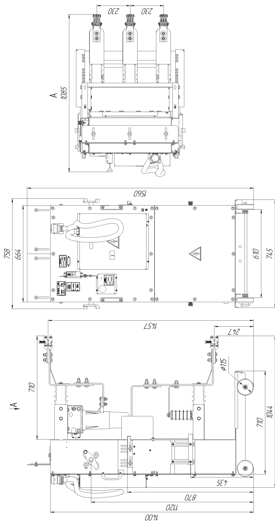
Рисунок Б.2 – Монтажный и габаритный чертеж выкатного элемента КЭПС-ВЭ КРУ 2-10 (вал вверх) с БУ
