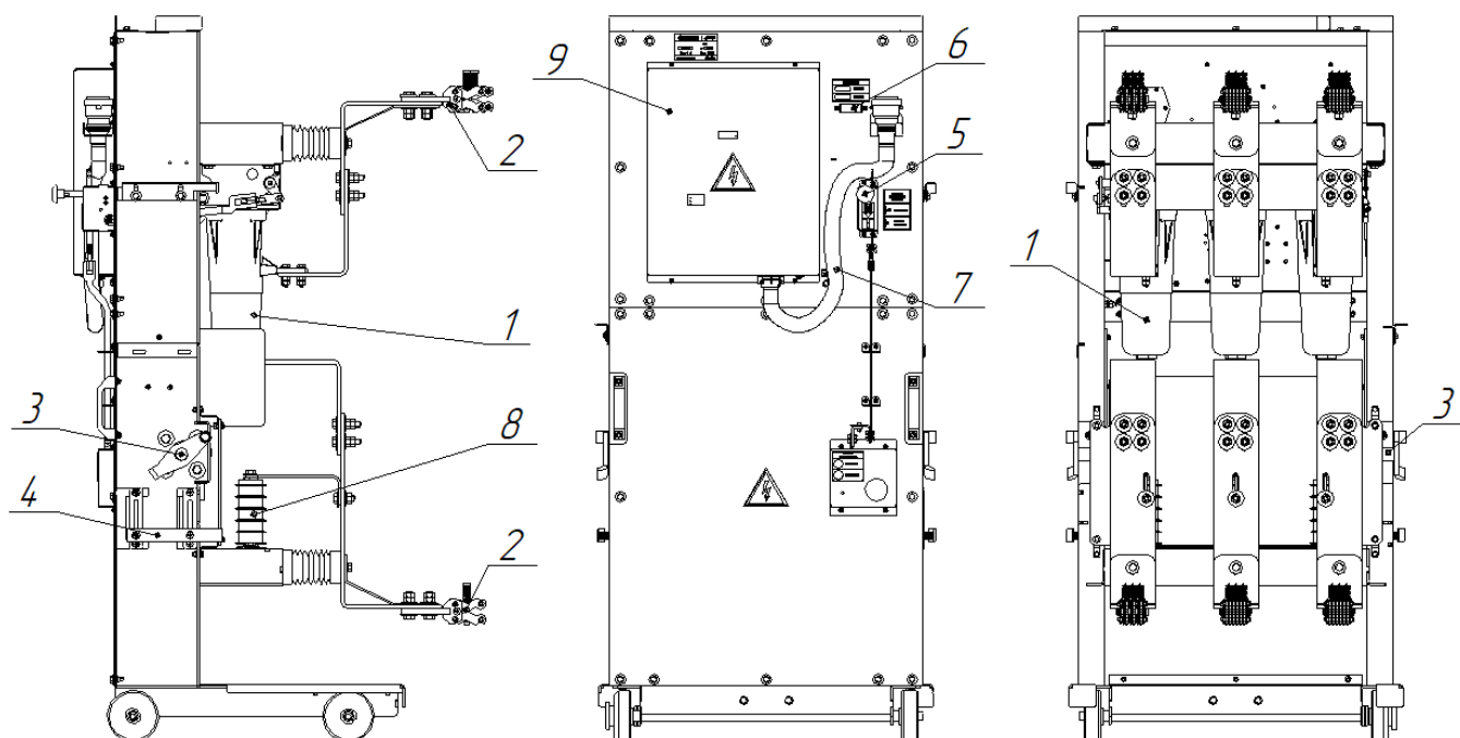
Рисунок 2.1 – Состав выкатного элемента КЭПС-ВЭ КРУ2-10 (КВЭ-10) вал вниз с БУ на щите
