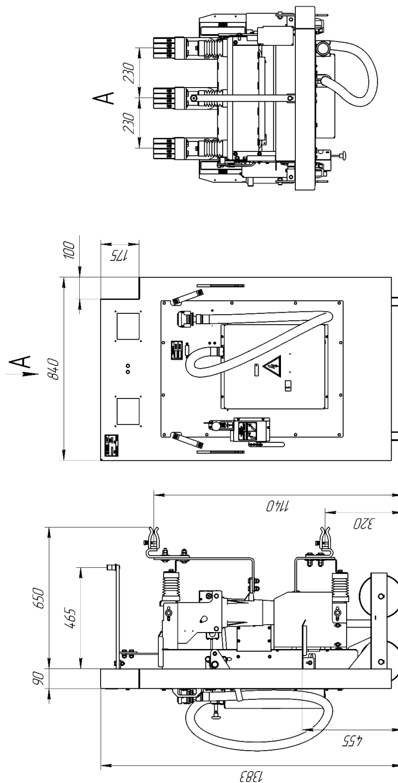
Рисунок А.1 – Габаритный чертеж выкатного элемента КЭПС-ВЭ К-XXVI 1000А с блоком управления на выкатном элементе
