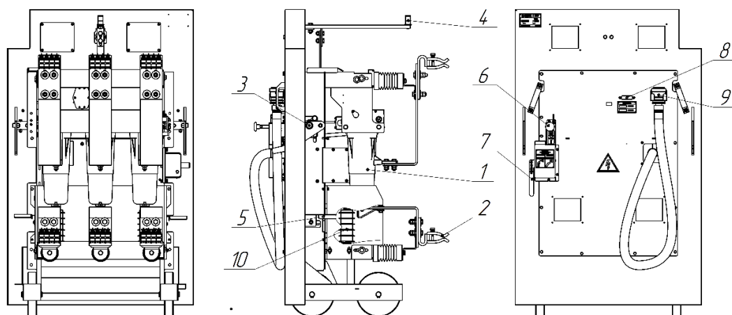
Рисунок 1 – Состав выкатного элемента без блока управления
