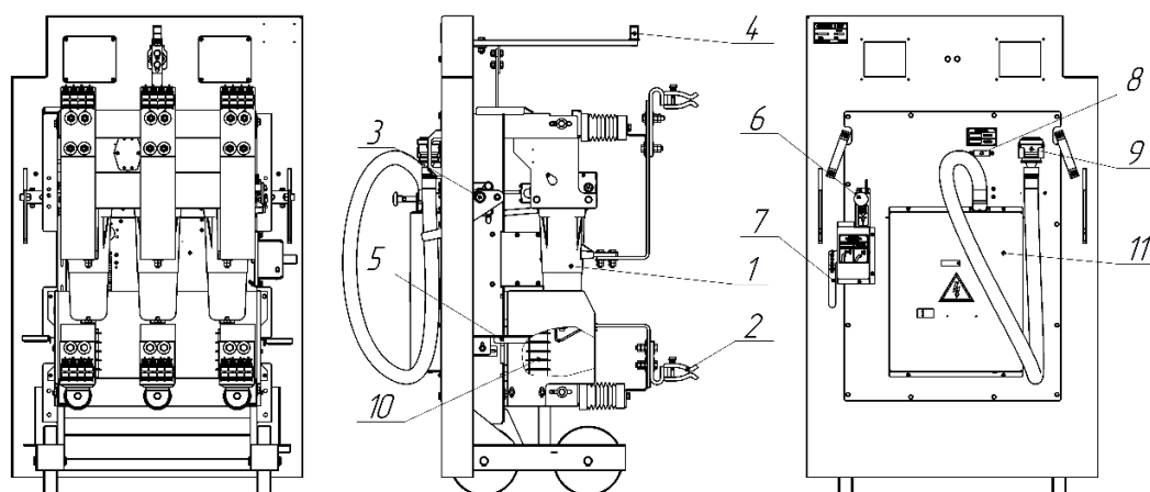
Рисунок 2 – Состав выкатного элемента с блоком управления
